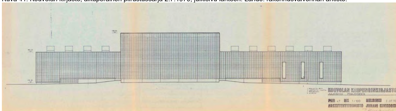
Kuva 42. Kouvolan kirjasto, alkuperäinen piirustussarja 2.7.1970, julkisivu pohjoiseen. Lähde: rakennusvalvonnan arkisto.
