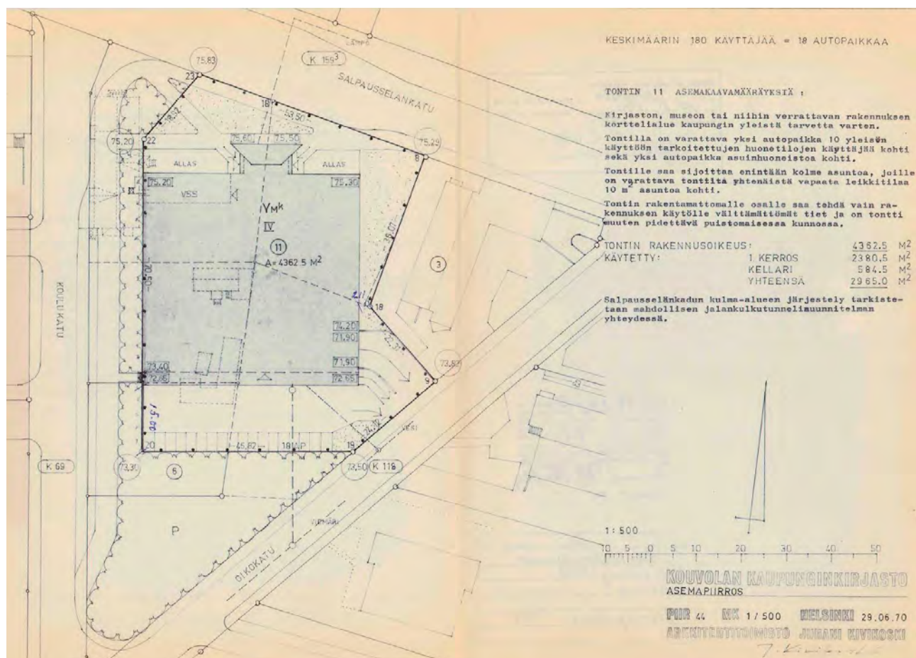
Kuva 38. Kouvola kirjasto, alkuperäinen, rakennusluvan yhteydessä ollut piirustussarja, piirustuksen päiväys 29.6.1970, Asemapiirustus ja asemakaavamääräykset. Lähde: rakennusvalvonnan arkisto.
